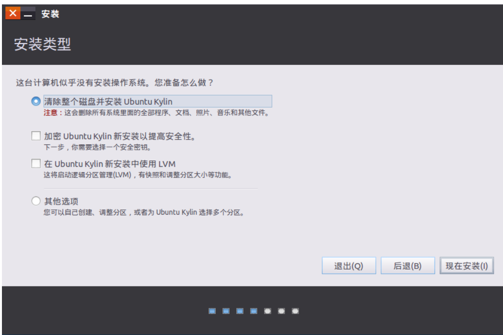
图 10 安装类型
