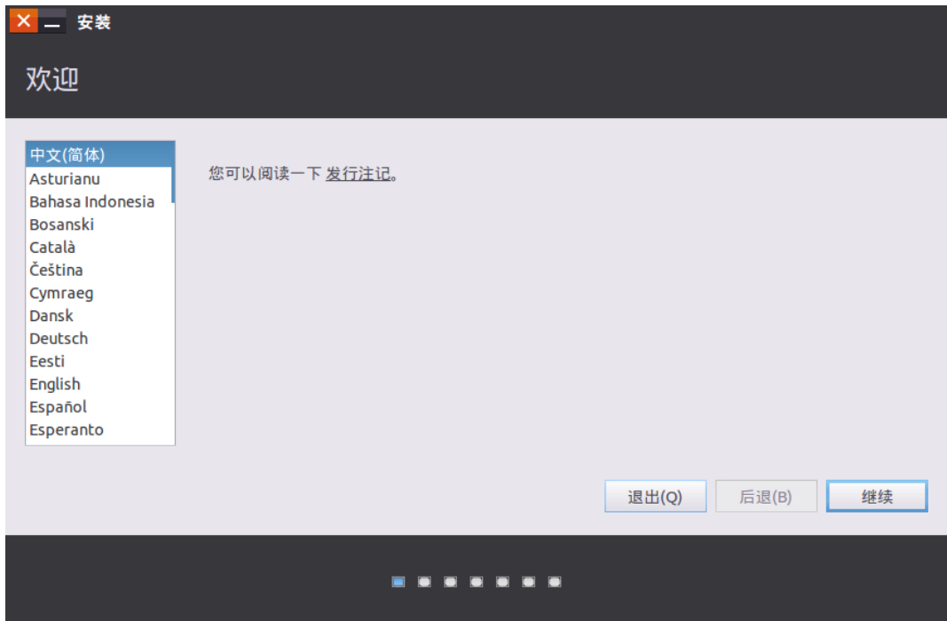
图 8 选择语言
