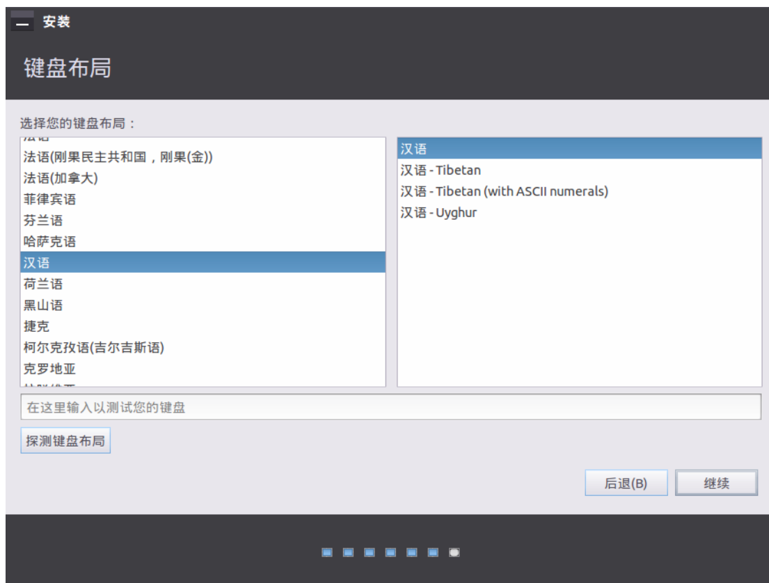
图 13 键盘布局
