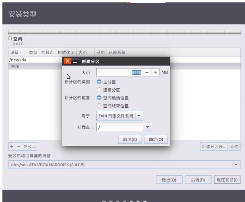
图 11 分区界面
